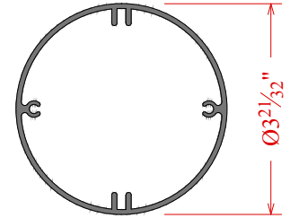
218-3 Rd. Post C7F5288
