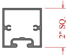
225 Std. Post C7G0288
