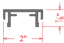
225 Std T/B Frame C6G01153
