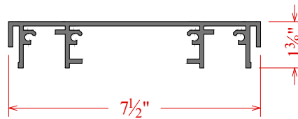
750 Std. T/B Frame C6L01219
