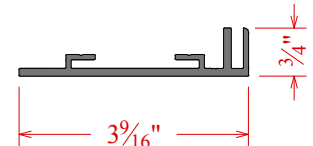
4000 T/B Frame C6Q41240
