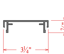
325 Std. T/B Frame C6K01153
